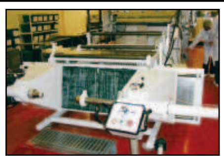
Beck Shaftless Unwind
