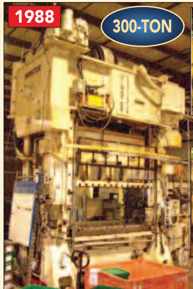
MINSTER 300 TON SSDC PRESS, MDL. E2-300-84-48
