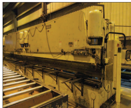
(2) Pacific 225 Ton x 13' CNC Hyd. Press Brakes
